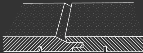
11. Profil chalet avec recouvrement de 3.5 mm 11. Chaletschalung mit Überdeckung 3.5 mm
