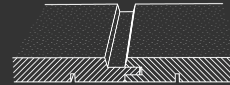
8. Profil canadien, ouv. 7 ou 11 mm 8. Schattennutprofil, Öff. 7 od. 11 mm
