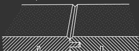
5. Profil chanfrein 5. Fastäfer
