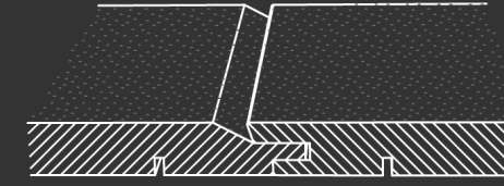
11.a Profil chalet avec recouvrement arrondi de 3.5 mm 11.a Chaletschalung mit gerundeter Überdeckung 3.5 mm
