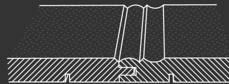
14. Profil doucine 14. Profil "doucine"
