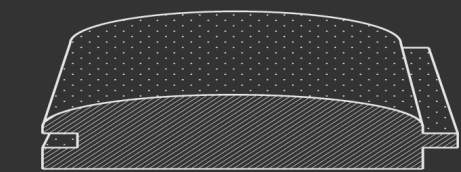
19. rainé-crête bombé 19. Gewölbt mit Nut und Kamm
