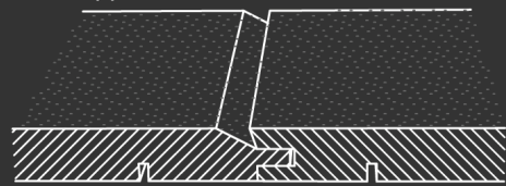
10. Profil chalet sans recouvrement 10. Chaletschalung ohne Überdeckung
