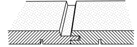
8. Profil canadien, ouv. 7 ou 11 mm 8. Schattennutprofil, Öff. 7 od. 11 mm
