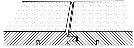
7. Profil en V 7. Steilfas
