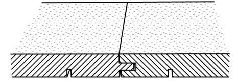
4. Profil plancher 4. Bodenriemen
