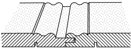
12. Profil antique, ouv 11 ou 14 mm 12. Landhaustäfer, Öff. 11 od. 14 mm
