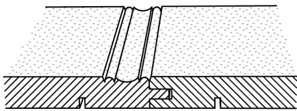
16. Profil griffes de chat sans ouverture 16. Katzenkrallentäfer ohne Öffnung
