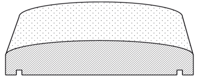
18. Bombé avec goutte pendante 18. Gewölbt mit anhängiger Tropfen
