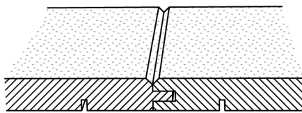
5. Profil chanfrein 5. Fastäfer
