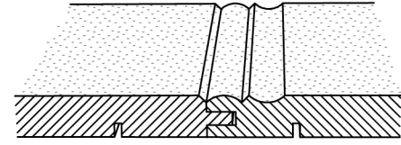
14. Profil doucine 14. Profil "doucine"
