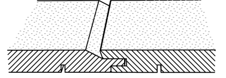
11.a Profil chalet avec recouvrement arrondi de 3.5 mm 11.a Chaletschalung mit gerundeter Überdeckung 3.5 mm
