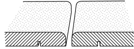
3. Raboté 3 faces angles arrondis 3. Glattkantprofil gerundet
