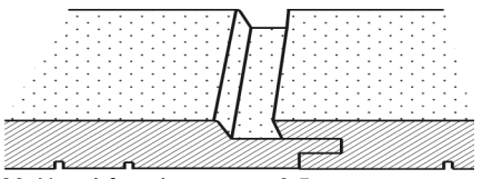
20. Ajouré fermé avec rec. 3.5 mm 20. Rhombo-geschlossen mit Überd. 3.5 mm
