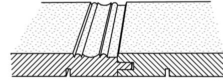
17. Profil griffes de chat, ouv. 3 ou 11 mm 17. Katzenkrallentäfer, Öff. 3 od. 11 mm
