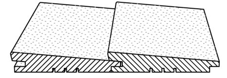
15. Trapézoïdal avec rec. 4.5 mm 15. Stülpchalung mit Überdeckung 4.5 mm
