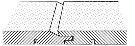
11. Profil chalet avec recouvrement de 3.5 mm 11. Chaletschalung mit Überdeckung 3.5 mm
