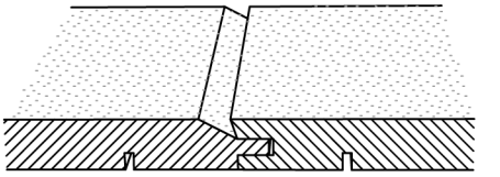
10. Profil chalet sans recouvrement 10. Chaletschalung ohne Überdeckung
